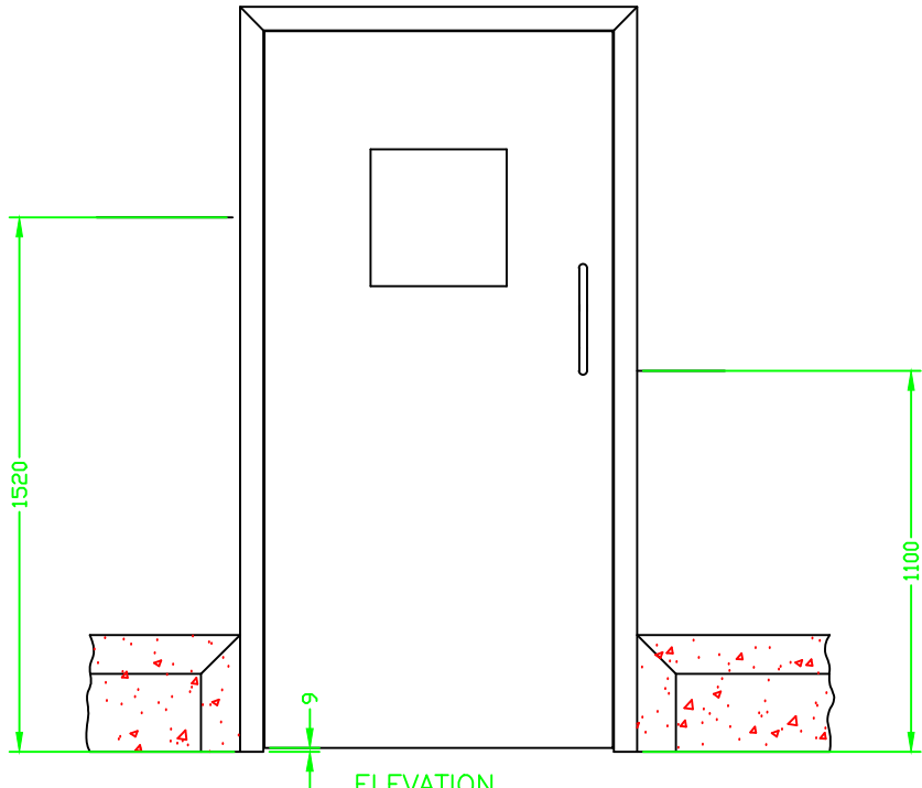
ELEVATION
