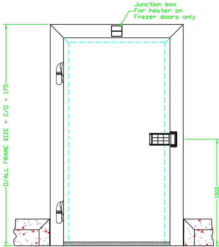
ELEVATION
