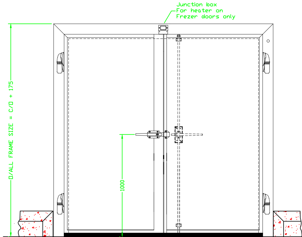
ELEVATION
